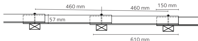
Længdesnit
