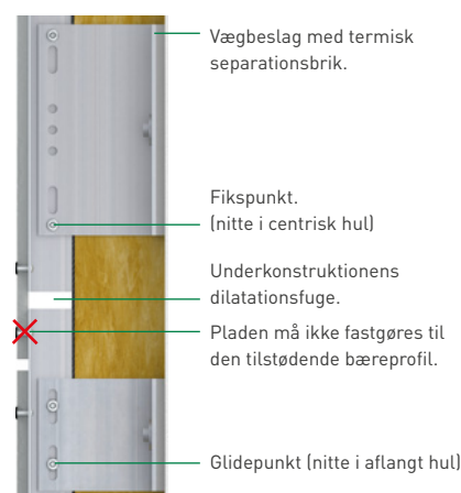
Detailsnit A: Etablering af aluminiumsunderkonstruktionens fikspunkter og glidepunkt.
