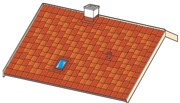
Figur 11. De mørkt markerede tagsten fastgøres altid. På steder med særlig belastning samt vind- og vejrforhold bindes samtlige sten.
