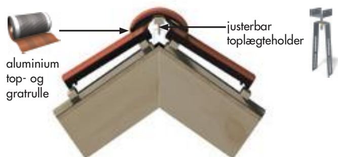
Figur 13. Anvendelse af Benders aluminium top- og gratrulle. Let at montere, skal blot ruller ud over toplægten, og lægges ned over de øverste rækker tagsten, hvorefter beskyttelsepapiret fjernes og rullen presses ned i tagstenens bølger.
