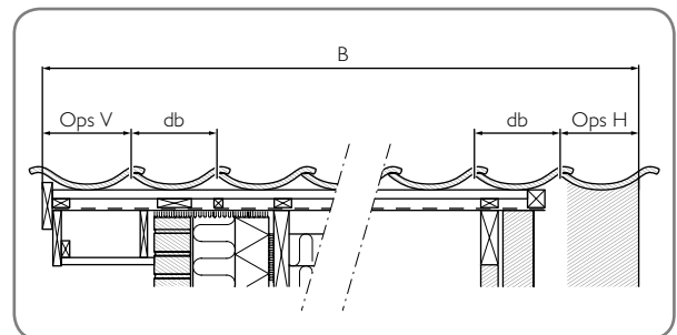
Gavl med dobbeltvinget tagsten
